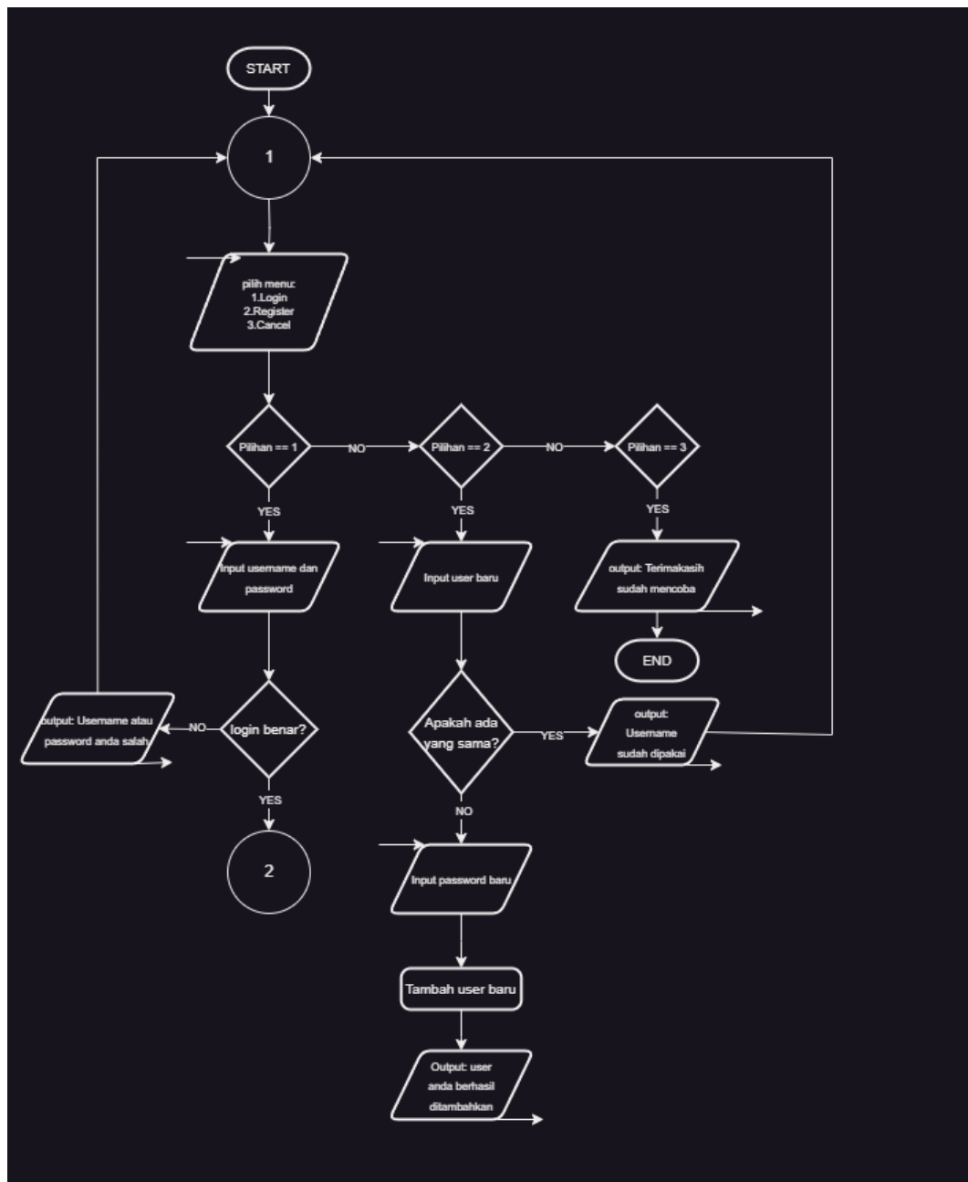
Flowchart menu utama
